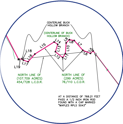
DETAIL "A" SCALE: 1" = 200'
